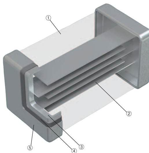
图1 层叠芯片变阻器的内部结构
