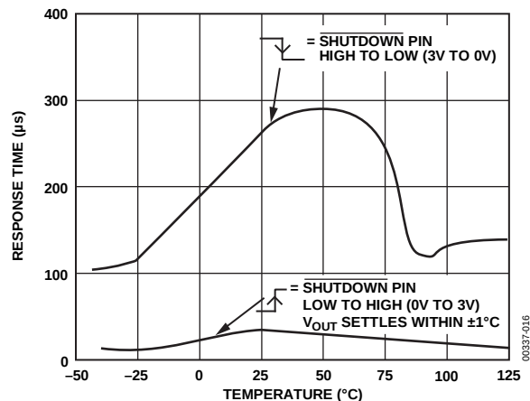
图15. \overline{\text{SHUTDOWN}} 引脚的 V_{OUT} 响应时间与温度的关系
