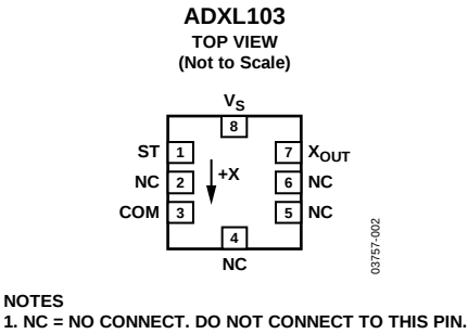
图3. ADXL103引脚配置
