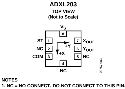
图4. ADXL203引脚配置
